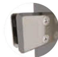
Pince inox pour vitrage verre feuilleté trempé 44/2 ép. 8.76 mm
