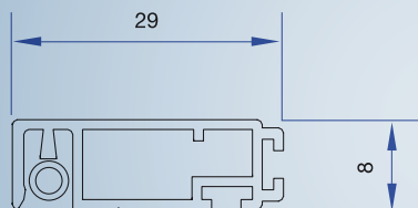
Section du cadre
